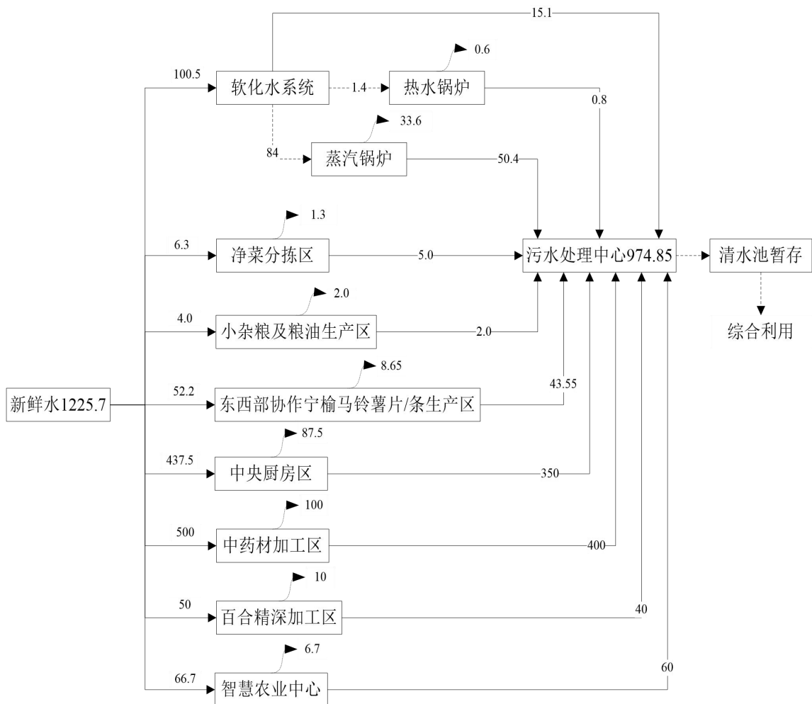
图 3.6.1 项目一期工程（采暖期）用水平衡图 单位：m³/d
