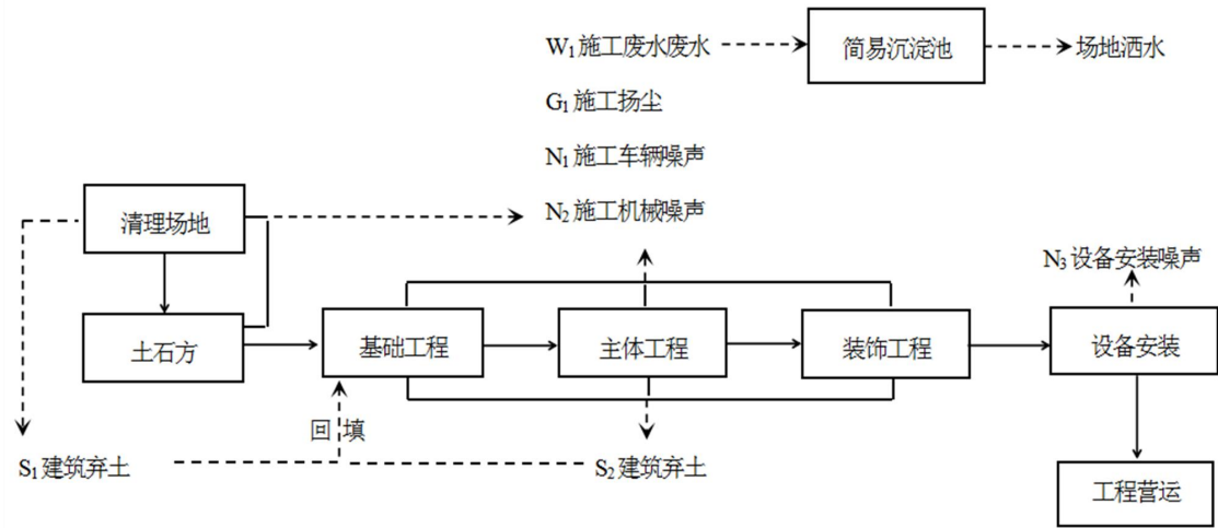
图 3.7-1 项目施工期工艺流程及产污节点图
