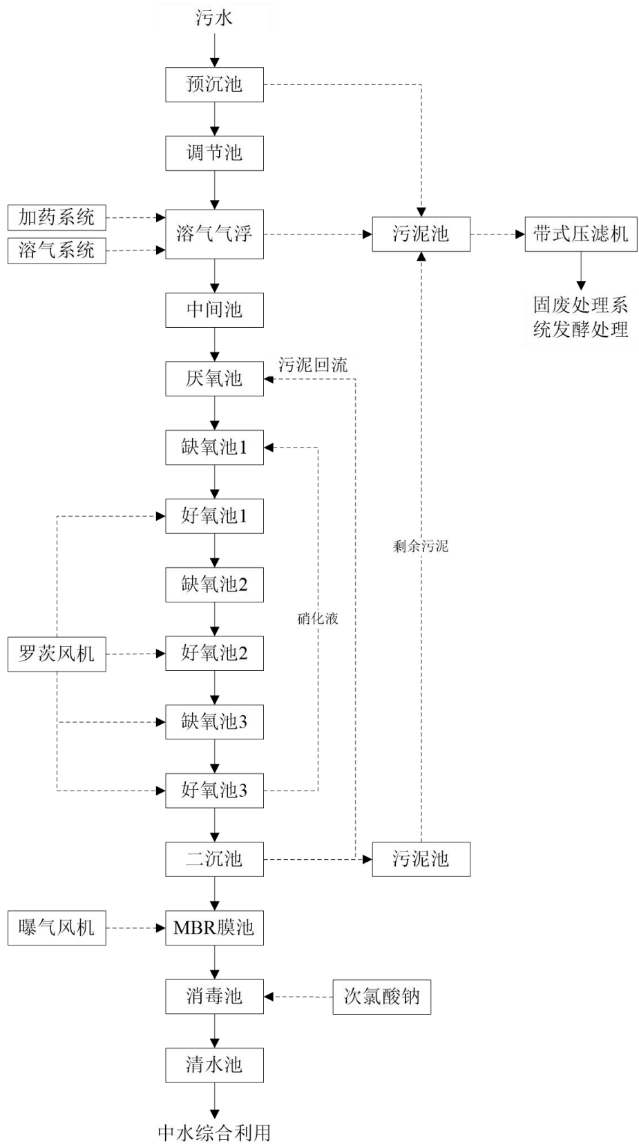
图 3.7-2 污水处理中心运行工艺流程及产污节点
