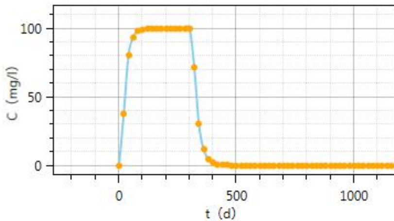
泄漏后入渗的废水对厂界氨氮贡献浓度-时间曲线
