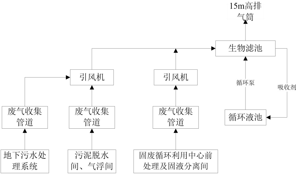
图 8.2-1 除臭系统流程图
