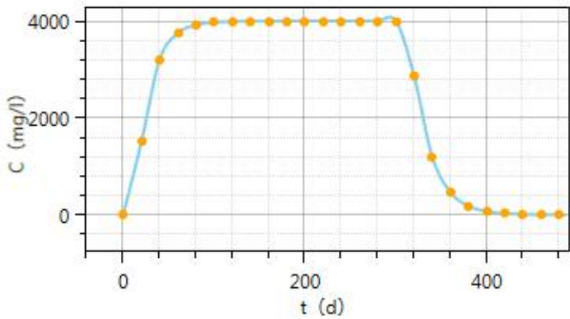
泄漏后入渗的废水对厂界 CODcr 贡献浓度-时间曲线
