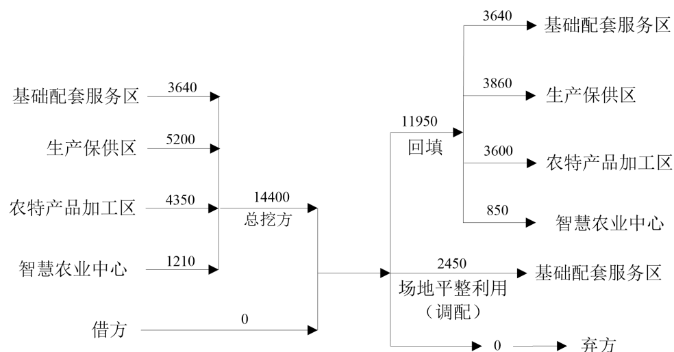
图 3.8-1 土石方流向平衡图 单位：m³
